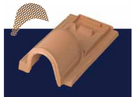
aeratore ad 1 tegola per marsigliese
